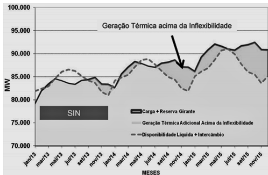
Figura 3 – Geração térmica acima da inflexibilidade, 2013-2015 (Soares, 2015 p.8)
