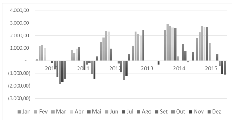
Figura 1 - Intercâmbio de energia N - SE/CO em MWmed, 2010-2015 (ONS, 2016 – Histórico de operação)
